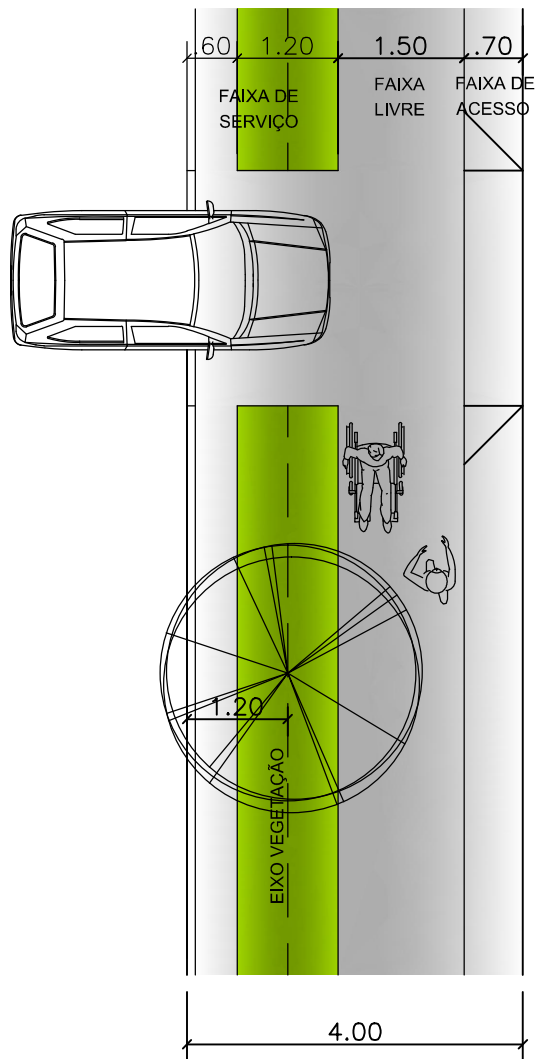
CALÇADA 4,00M PLANTA BAIXA
