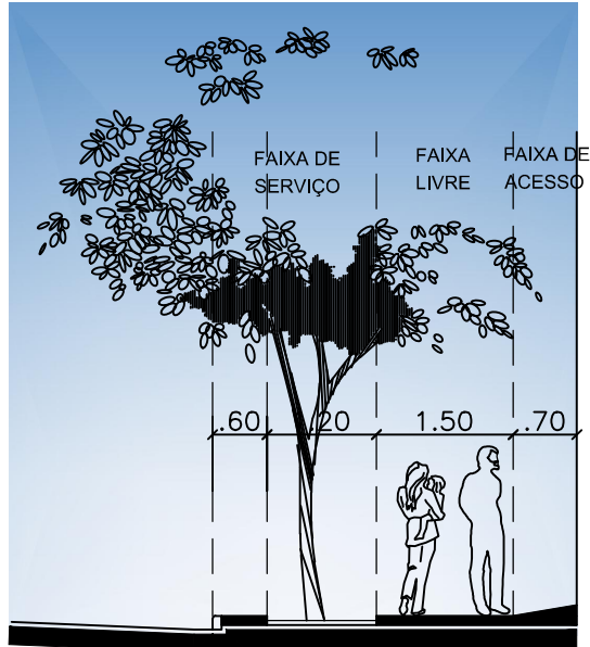
CALÇADA 4,00M CORTE
