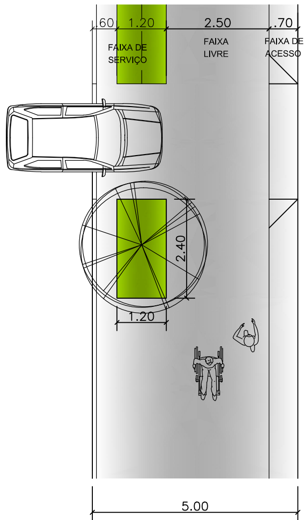
CALÇADA 5,00M PLANTA BAIXA
