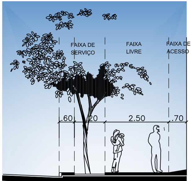
CALÇADA 5,00M CORTE
