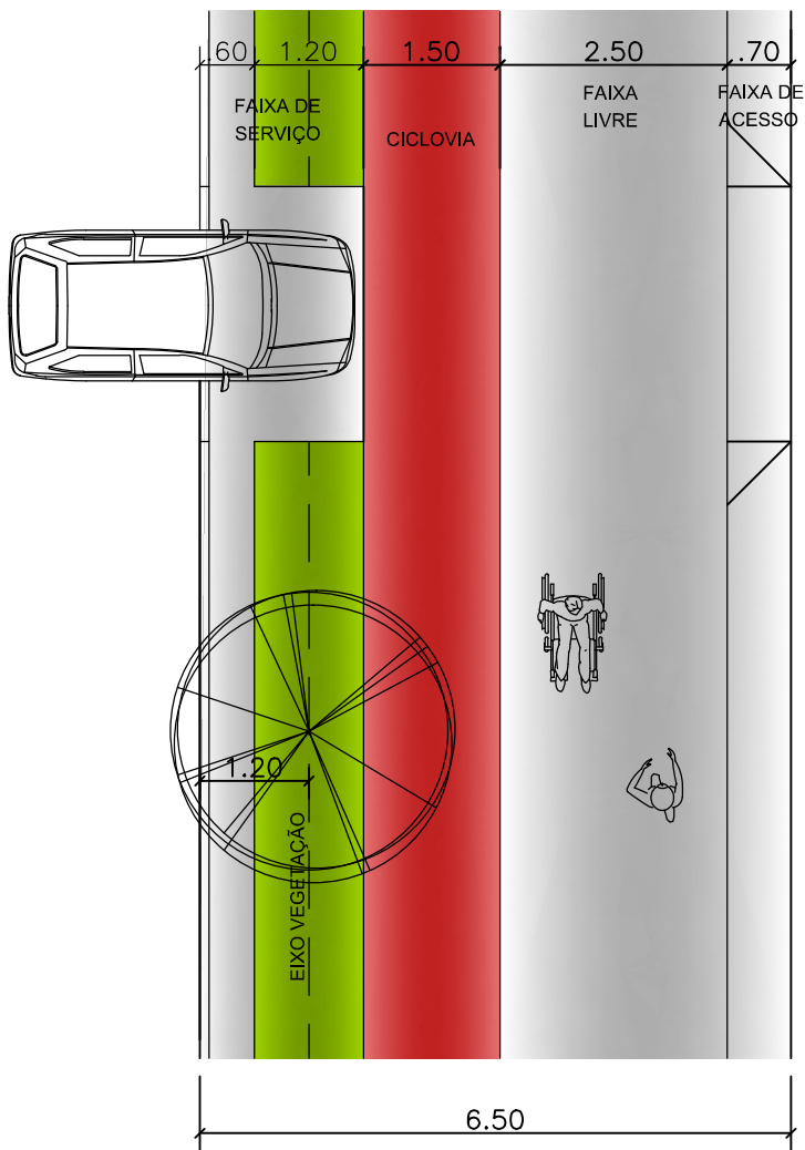
CALÇADA 6,50M PLANTA BAIXA
