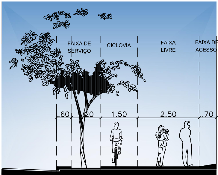
CALÇADA 6,50M CORTE
