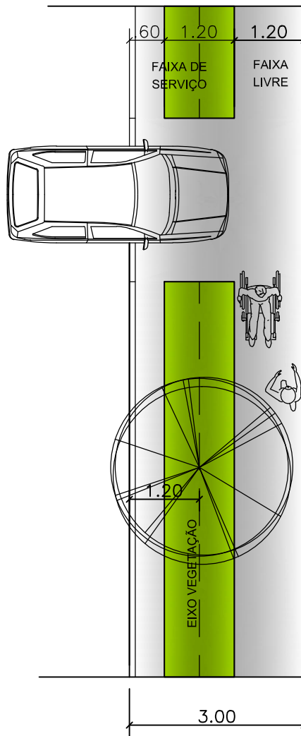
CALÇADA 3,00M PLANTA BAIXA
