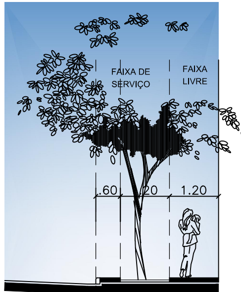
CALÇADA 3,00M CORTE
